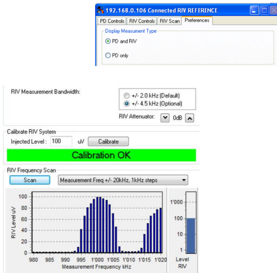
Сканирование частот для нахождения частоты без паразитных сигналов для измерения радиопомех
