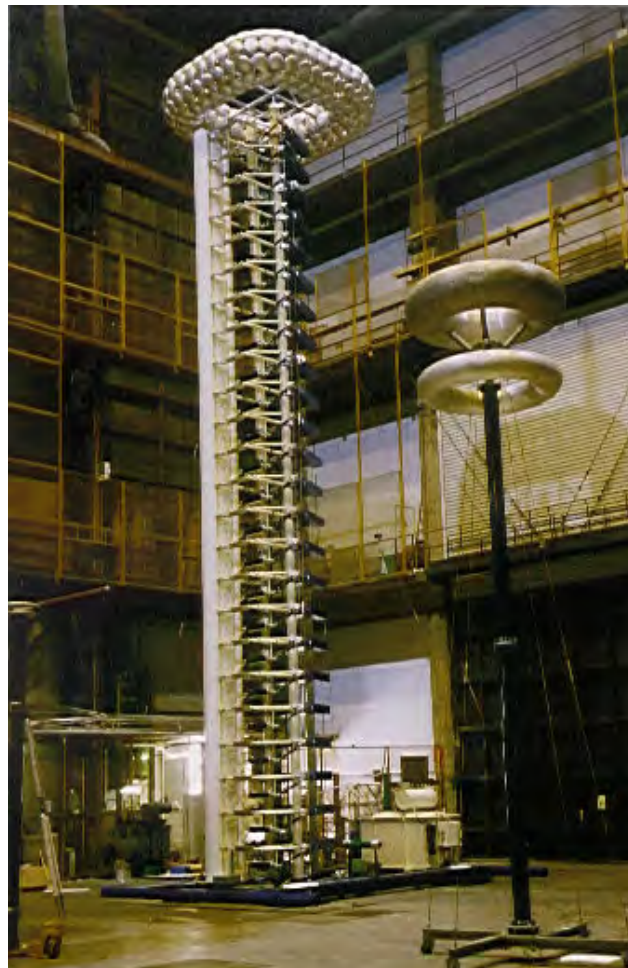
4800 kV impulse generator at CESI, Milano
